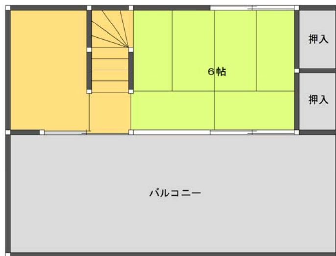
2階平面図
